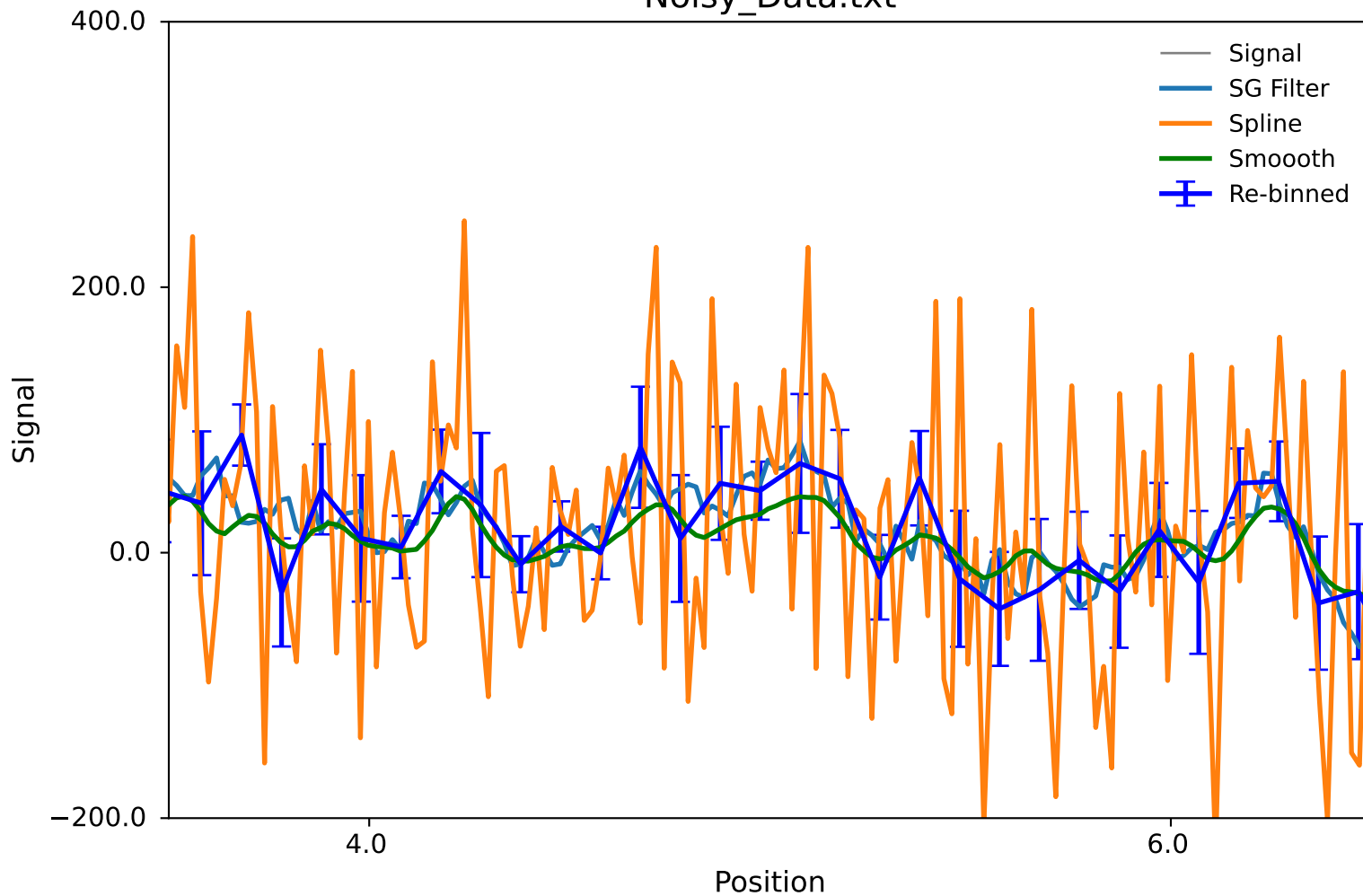
Noisy_Data.txt
