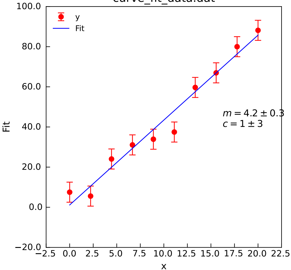
curve_fit_data.dat
